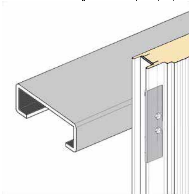
2-fache Verschraubung mit Lastverteilerplatte (LVP)
